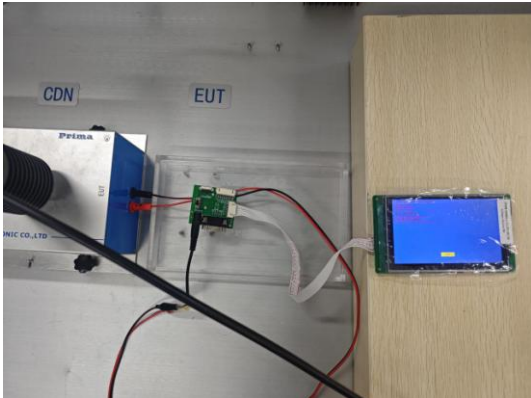
图 4-4 CS 测试图
