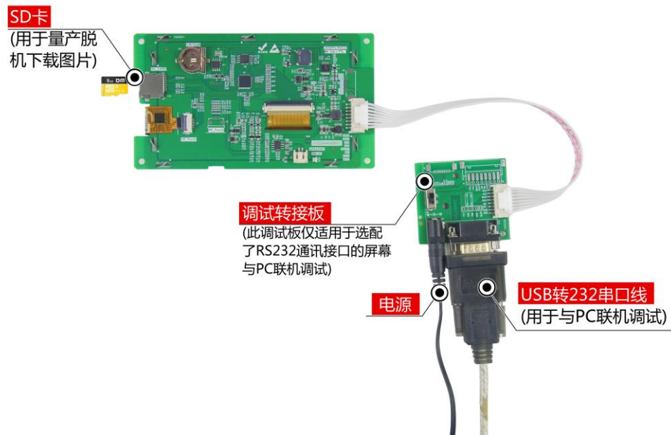
图 1-5 调试工具图
