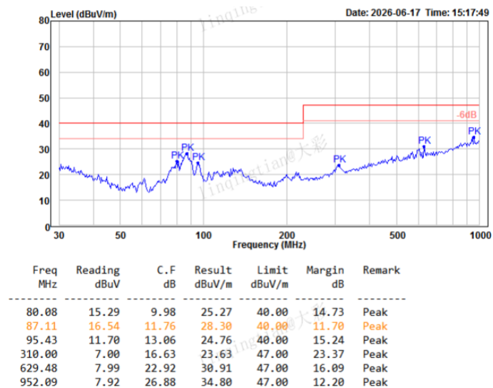
图 4-7 RE 测试垂直方向
