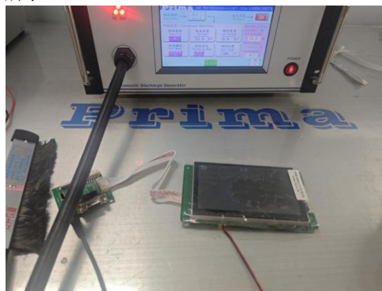
图 4-2 ESD 测试图
