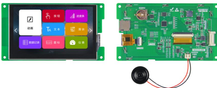
图 1-2 5.0 寸电容触摸参考图
