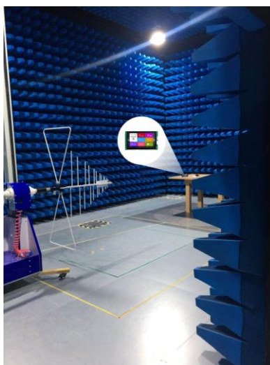
图 4-5 RE 测试图
