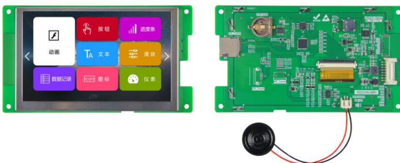
图 1-3 5.0 寸无触摸参考图
