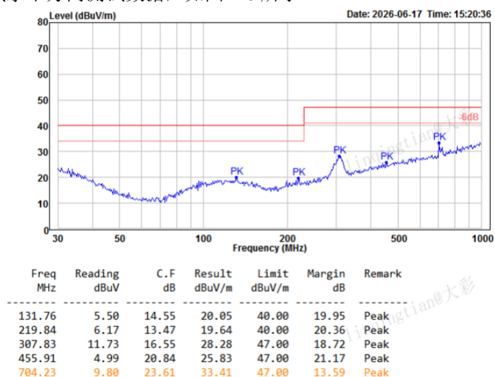
图 4-6 RE 测试水平方向
