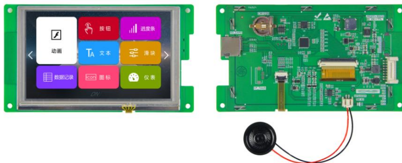
图 1-1 5.0 寸电阻触摸参考图
